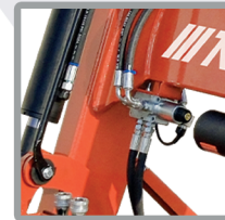
Hareketli Ataşman Valfi
